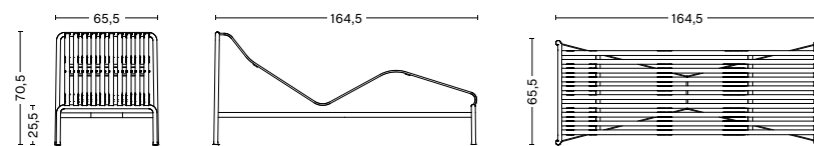
PALISSADE CHAISE LONGUE Width 65,5 cm Depth 164,5 cm Height 70,5 cm Seat height 25,5 cm
