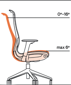
Keinun jäykkyyden säätö
